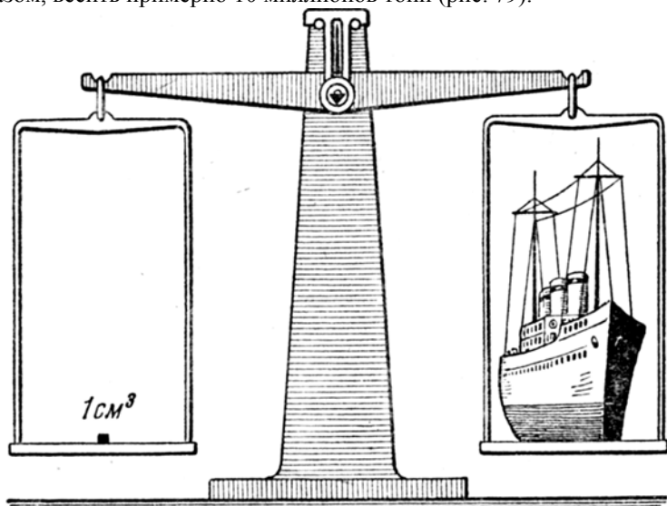
Рис. 79. Один кубический сантиметр атомных ядер мог бы уравновесить океанский пароход даже и при весьма неплотной упаковке их. Плотнo же уложенные в объёме 1 \text{ см}^3 атомные ядра весили бы 10 миллионов тонн!
