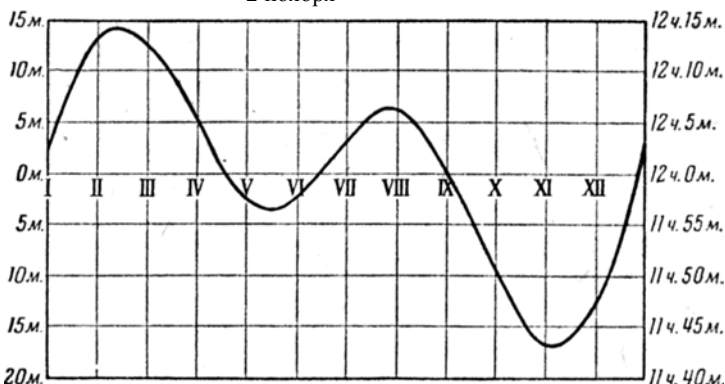
Рис. 7. Этот график, именуемый «графиком уравнения времени», показывает, как велико в тот или иной день расхождение между истинным и средним солнечным полуднем. Например, 1 апреля в истинный полдень верные механические часы должны показать 12 ч. 5 мин.; иными словами, кривая даёт среднее время в истинный полдень.
