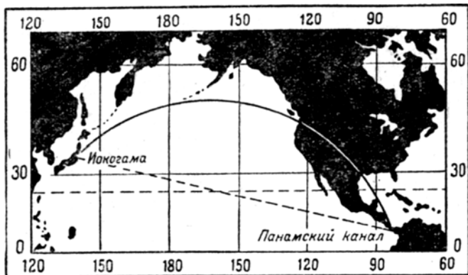
Рис. 2. Кажется невероятным, что криволинейный путь, соединяющий на морской карте Иокогаму с Панамским каналом, короче прямой линии, проведённой между теми же точками.
