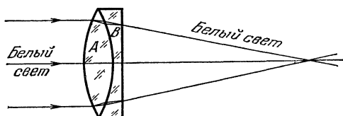
Рис. 17. Ахроматический объектив.
