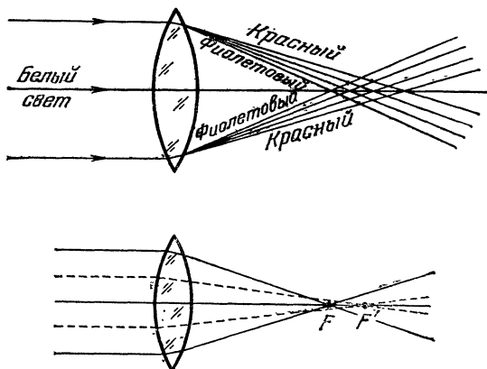
Рис. 14. Хроматическая (вверху) и сферическая абберации.
