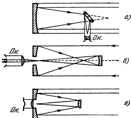
Рис. 21. Ход луча в рефракторах системы Ньютона (а), Грегори (б) и Кассегрена (в).
