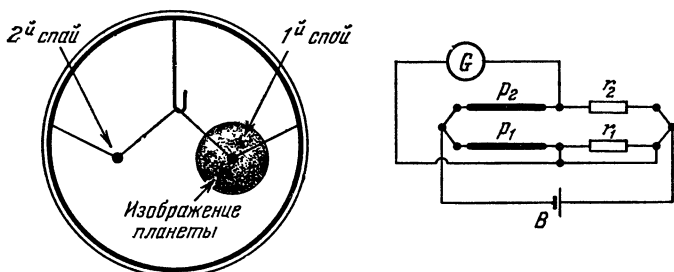
Рис. 38. Термоэлемент и болометр.
