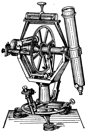
Рис. 30. Универсальный инструмент.
