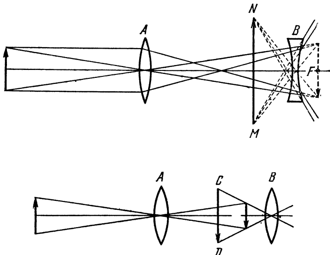
Рис. 13. Галилеевский (вверху) и кеплеровский телескопы (схема).
