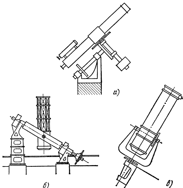
Рис 27. Типы установок (штативов) телескопов: немецкий (а), английский (б), американский (в).
