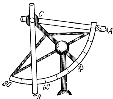
Рис. 5. Универсальный квадрант.
