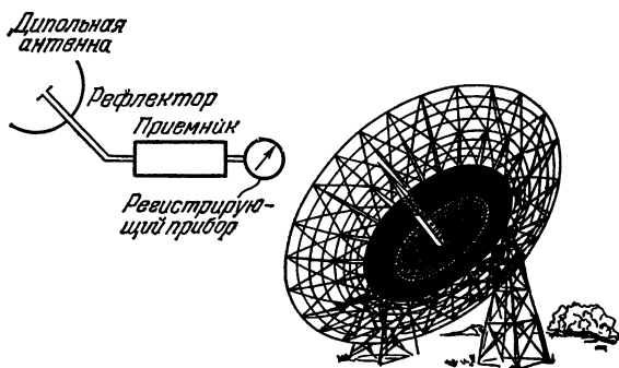
Рис. 40. Схема устройства радиотелескопа.
