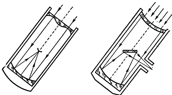
Рис. 26. Зеркально-линзовые системы Шмидта (слева) и Максудова.
