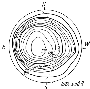
Рис. 43. Инфракрасная карта Венеры.
