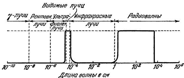
Рис. 39. Прозрачность земной атмосферы.
