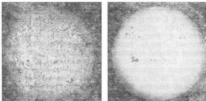
Рис. 37. Слева — спектрогелиограмма Солнца (в лучах водорода). Справа — обычный снимок Солнца.
