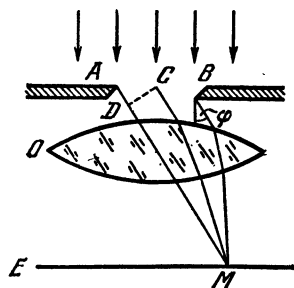
Рис. 36. Дифракция света от одной щели.
