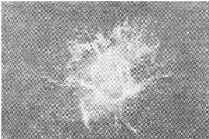
Рис. 45. Фотография Крабовидной туманности.
