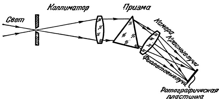
Рис. 33. Схема спектрографа.
