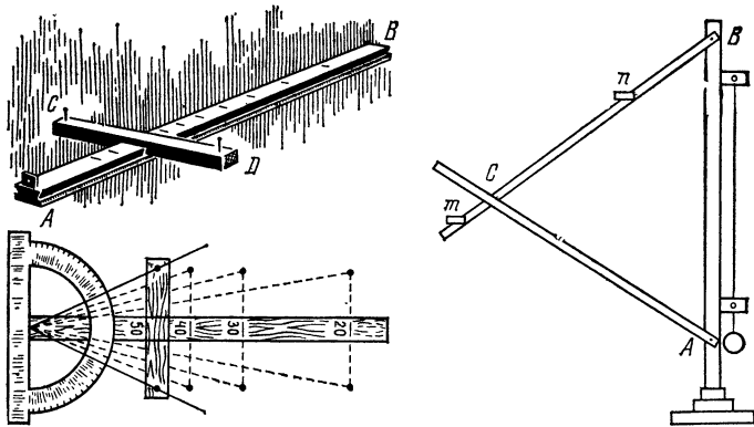
Рис. 2. Астрономический посох (слева вверху) и трикветр (справа). Слева внизу чертеж, поясняющий принцип действия астрономического посоха.
