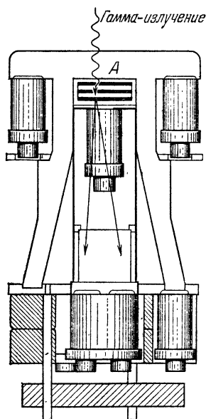
Рис. 44. Схема гамма-телескопа.
