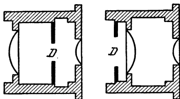
Рис. 18. Окуляры Гюйгенса (слева) и Рамсдена. D — диафрагма.
