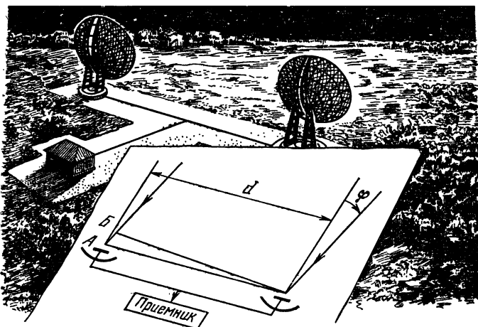
Рис. 41. Схема радиointерферометра ( d — его база, т. е. расстояние между радиотелескопами, угол \varphi характеризует направление на источник радиоволн).
